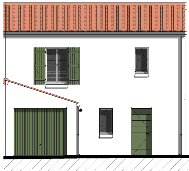
Façade Avant ( 1 : 100 )
